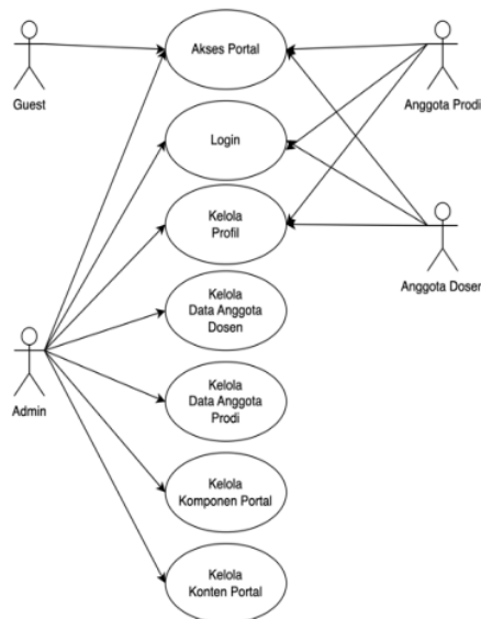
Gambar 2. Use Case sistem PIAUD
